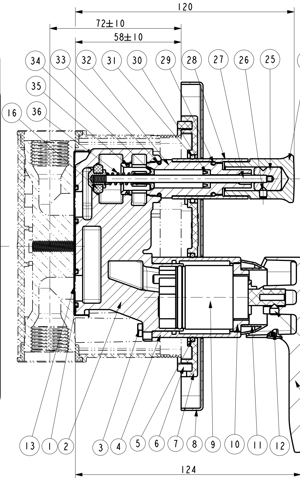
SECTION A-A
