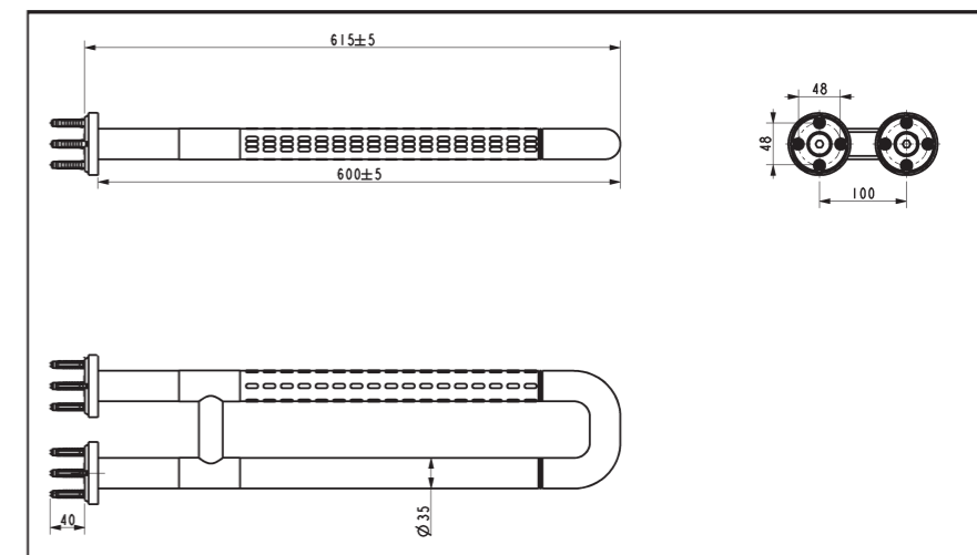
FFAS9402-000040BC0 (CF-9402.000.04) 部分尺寸图
