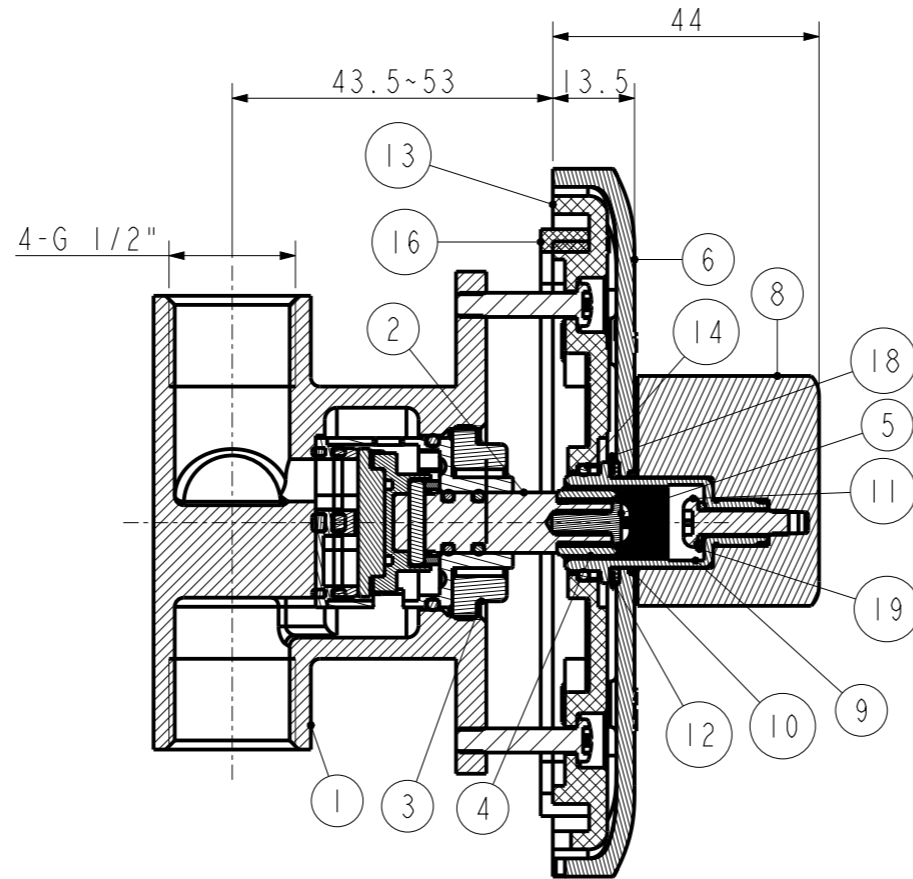
截面 A-A
