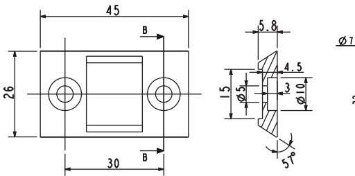
底座安装孔
